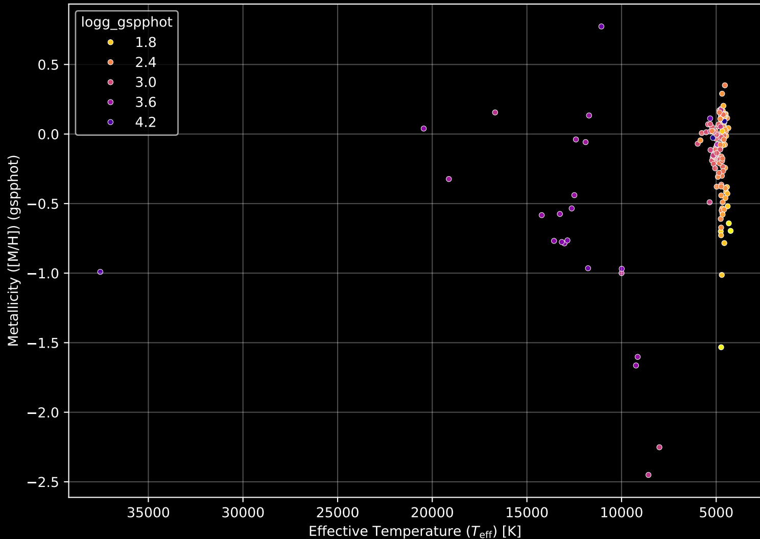
APOGEE DR17 Field: [101-04] Stellar Population Parameters (n= 158)
